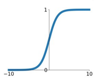
Sigmoid
