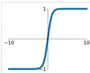
tanh
